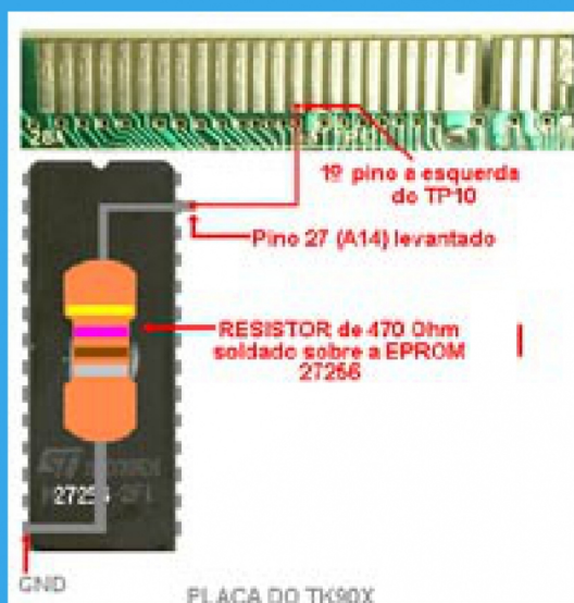
Figura 6: Ligações no TK90X
