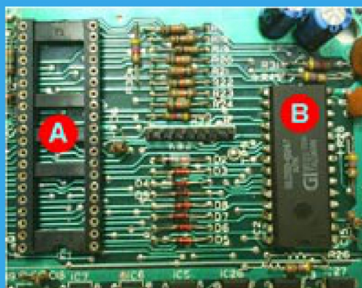
Figura 1: A) Soquete da ULA; B) ROM do TK90X.
