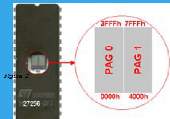
Figura 2: Uma EPROM 27256
