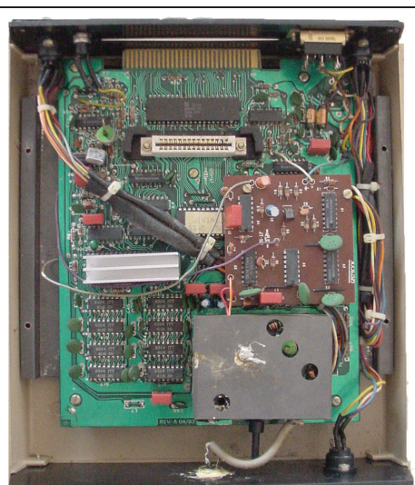
Fotos, gentilmente cedidas pelo Sr. Kazuaki, do protótipo do Splicevision.
