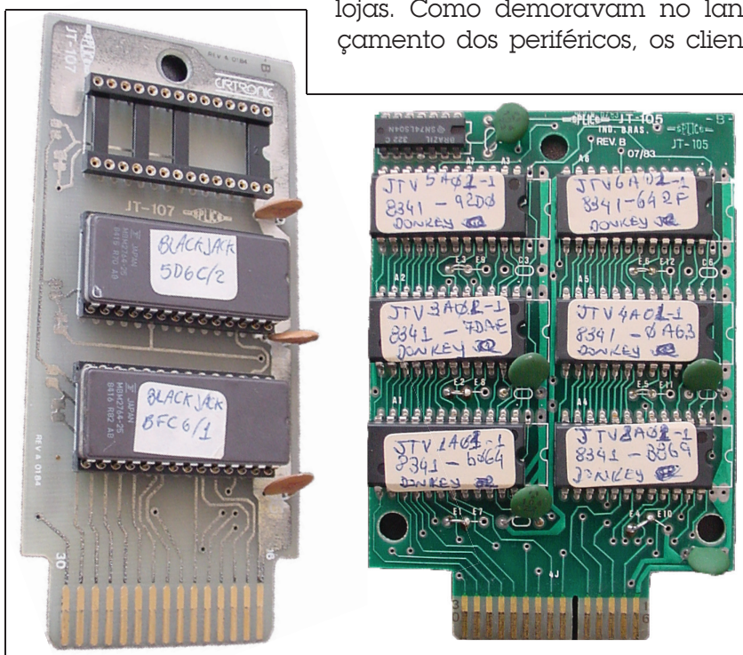
Acima, os dois tipos de placas dos cartuchos do Splicevision, utilizadas, uma ou outra, dependendo do jogo: à esquerda, modelo para até 3 EPROMs; à direita, placa para até 6 EPROMs.
