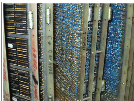
Fig.2: Assim eram os chips Agnus e Daphne (que se tornou Denise), em fase de protótipo. Note que foi usada a técnica de "wire-wrap" para conexão dos circuitos!
